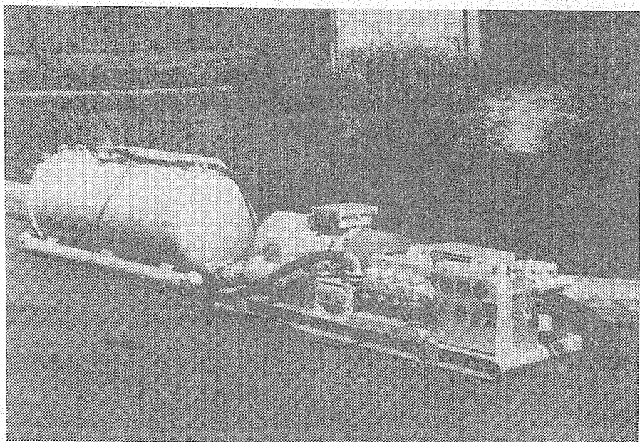
Výrobek oceněný zlatou medailí na Strojírenském veletrhu v Brně — hydraulický agregát HA 80/320.
