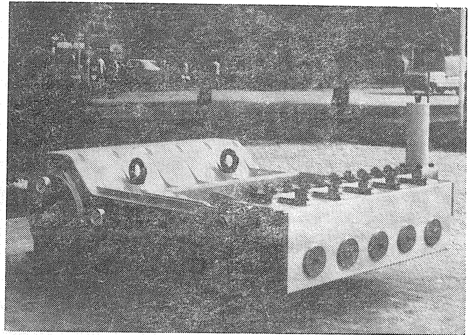
Vysokotlaké plunžrové čerpadlo PAH-5-140, výrobek k. p. Sigma Hranice, oceněné zlatou medailí na MSV Brno 1980
