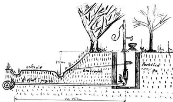
{Nákres vodovodu pod silnicí a čerpadla, v originálu proveden barevnými pastelkami.}
